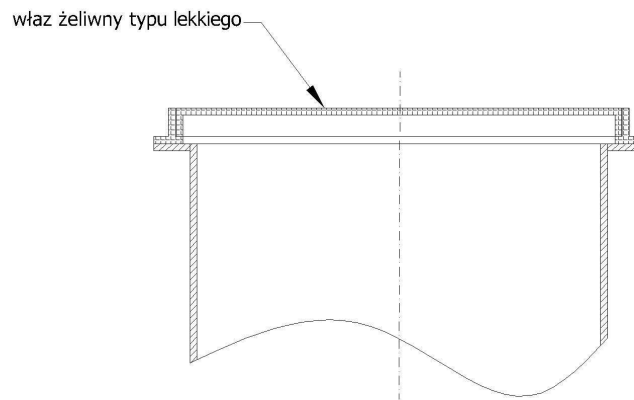
Zwieńczenie separatora włazem żelwnym typu lekkiego
