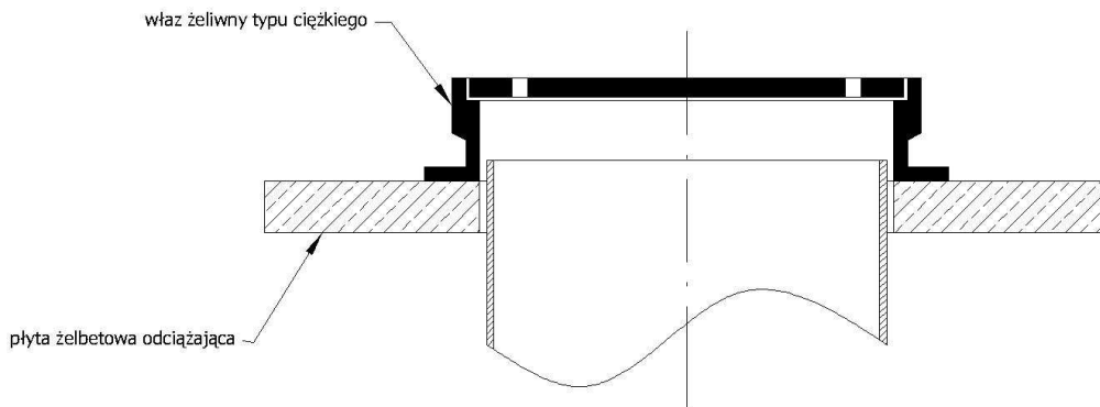
Zwieńczenie separatora włazem żelwnym typu ciężkiego
