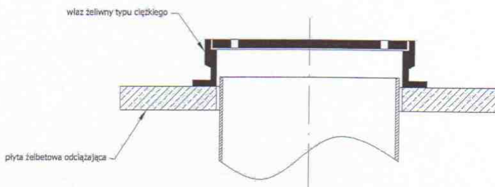
Zwienczenie separatora włazem żeliwnym typu ciężkiego
