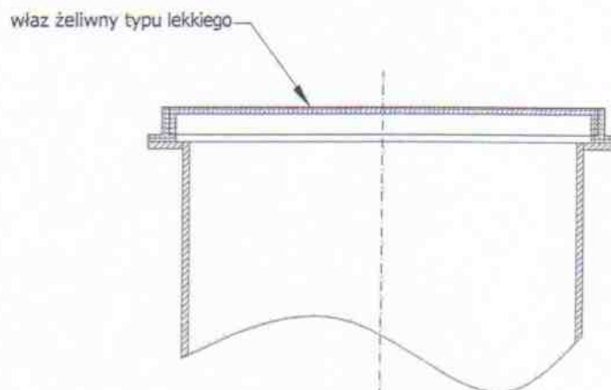
Zwienczenie separatora włazem żeliwnym typu lekkiego
