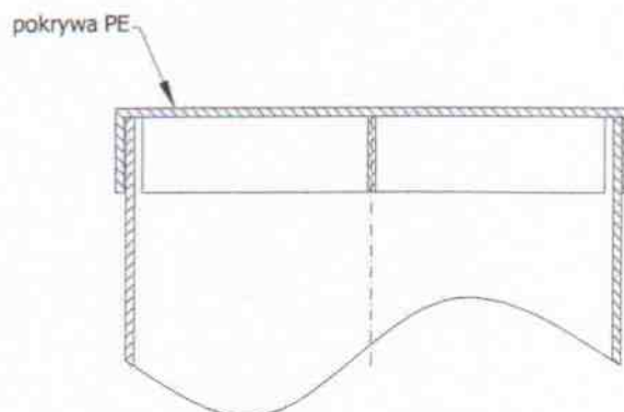
Zwienczenie separatora włazem z tworzywa sztucznego (PEHD)
