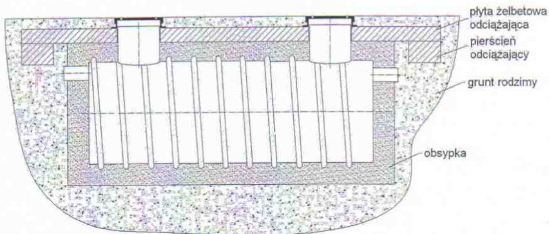
Montaż separatora w terenie najazdowym
