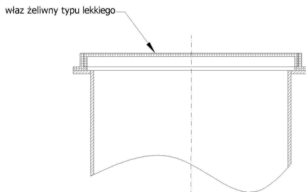
Zwieńczenie studzienki włazem żeliwnym typu lekkiego
