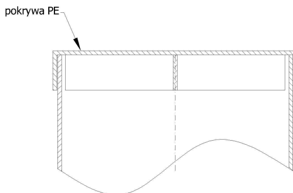
Zwieńczenie studzienki wężem z tworzywa sztucznego (PEHD)
